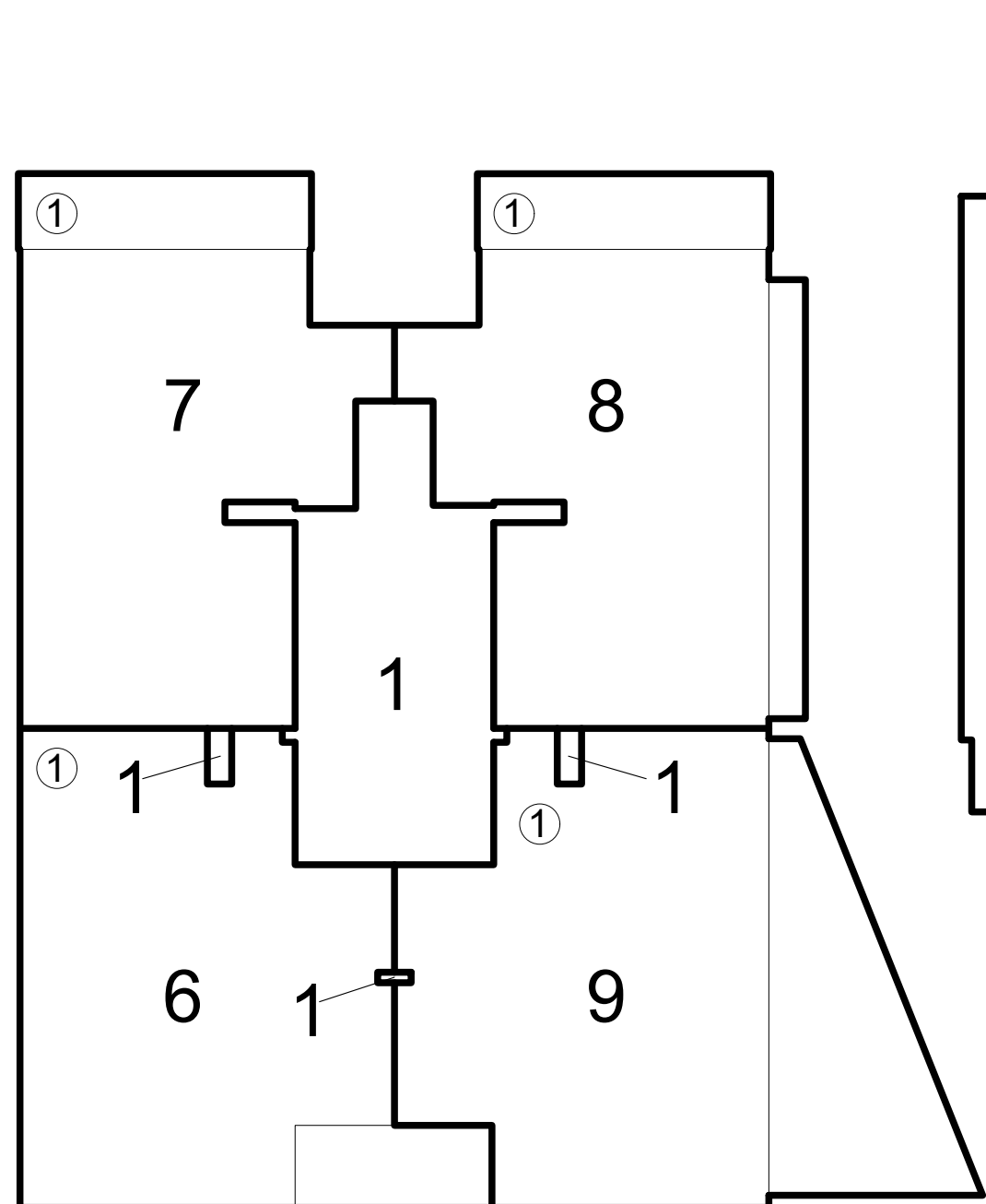
1 e verdieping Blok A 0m 2m 10m Schaal 1:200
