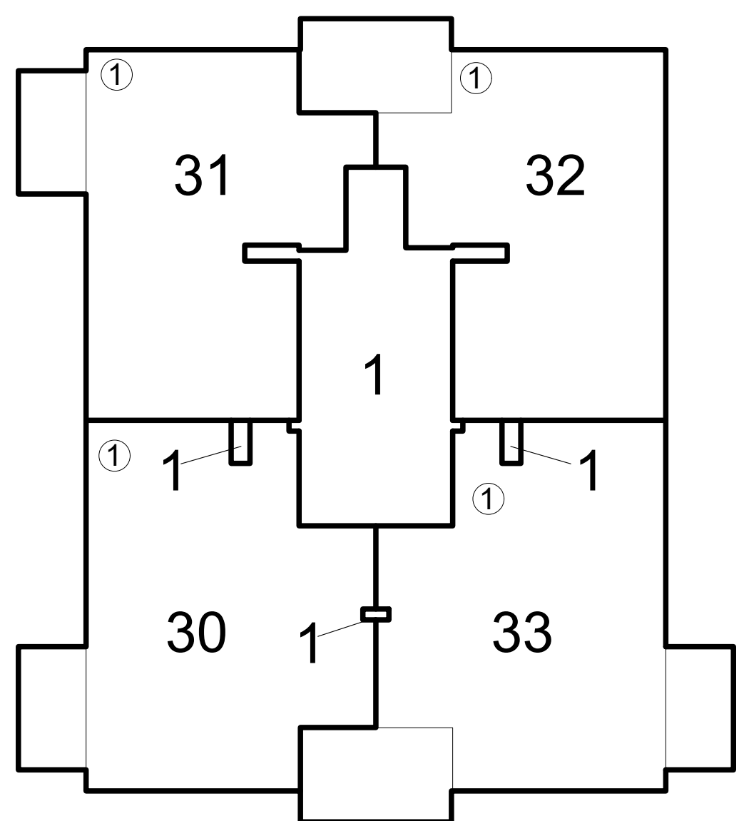
7 e verdieping Blok A 0m 2m 10m Schaal 1:200
