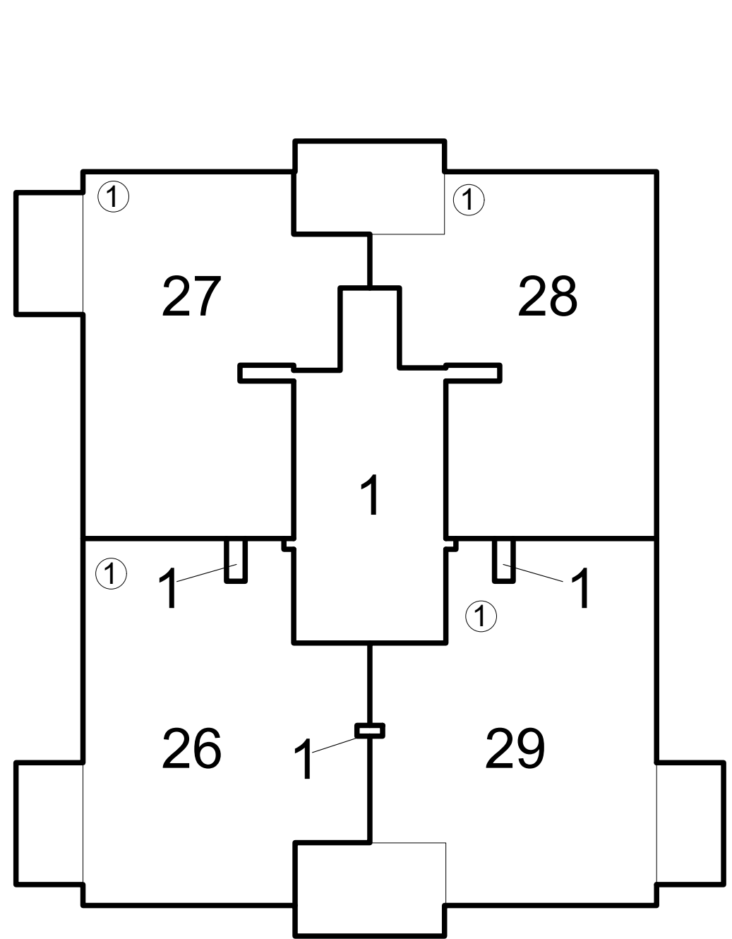
6 e verdieping Blok A 0m 2m 10m Schaal 1:200
